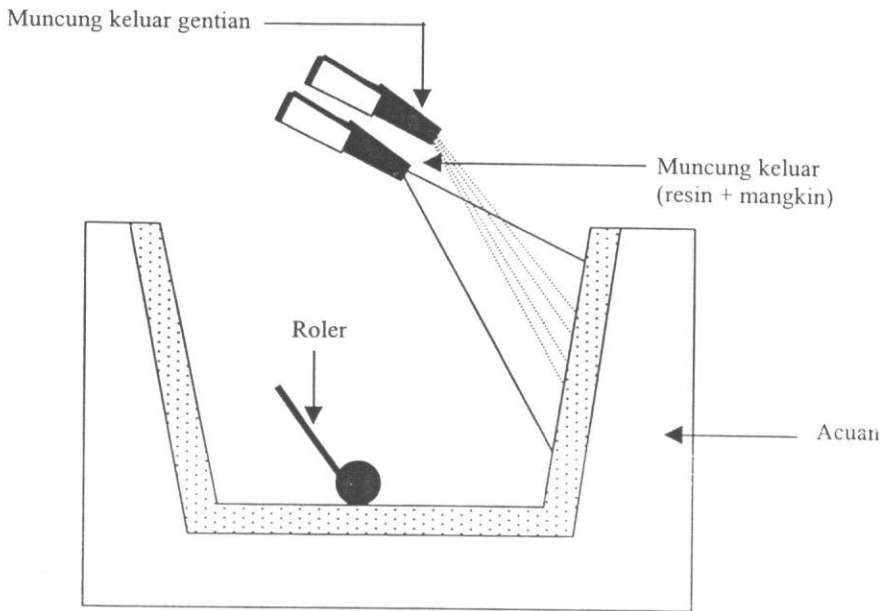
Rajah 2 Kaedah Asas Semburan
