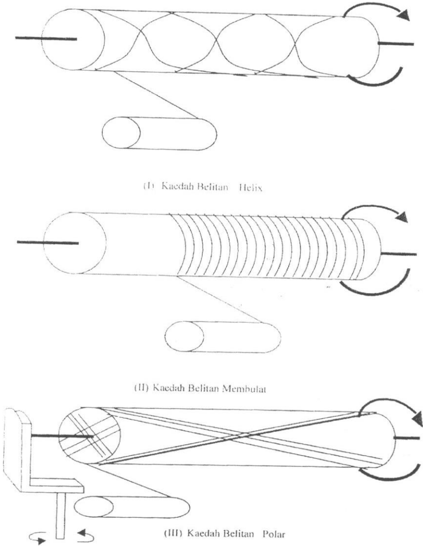
Rajah 5 Teknik-Teknik Belitan
