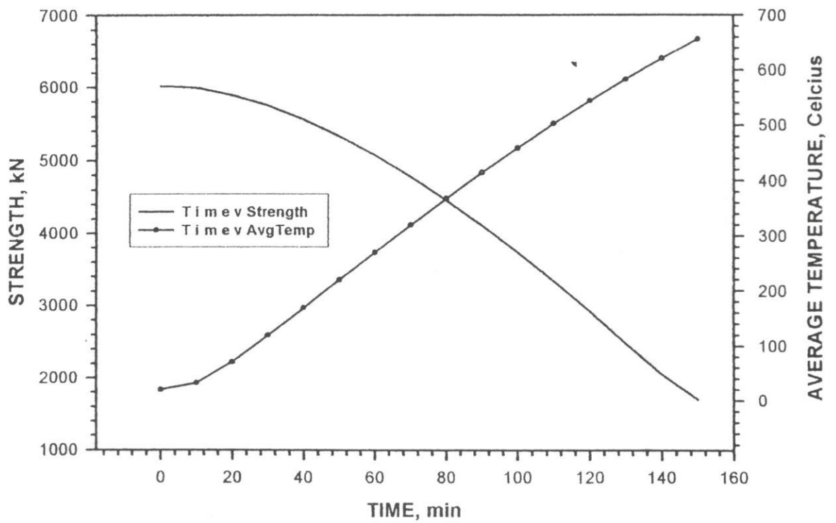
Fig. 14 Column FS3
