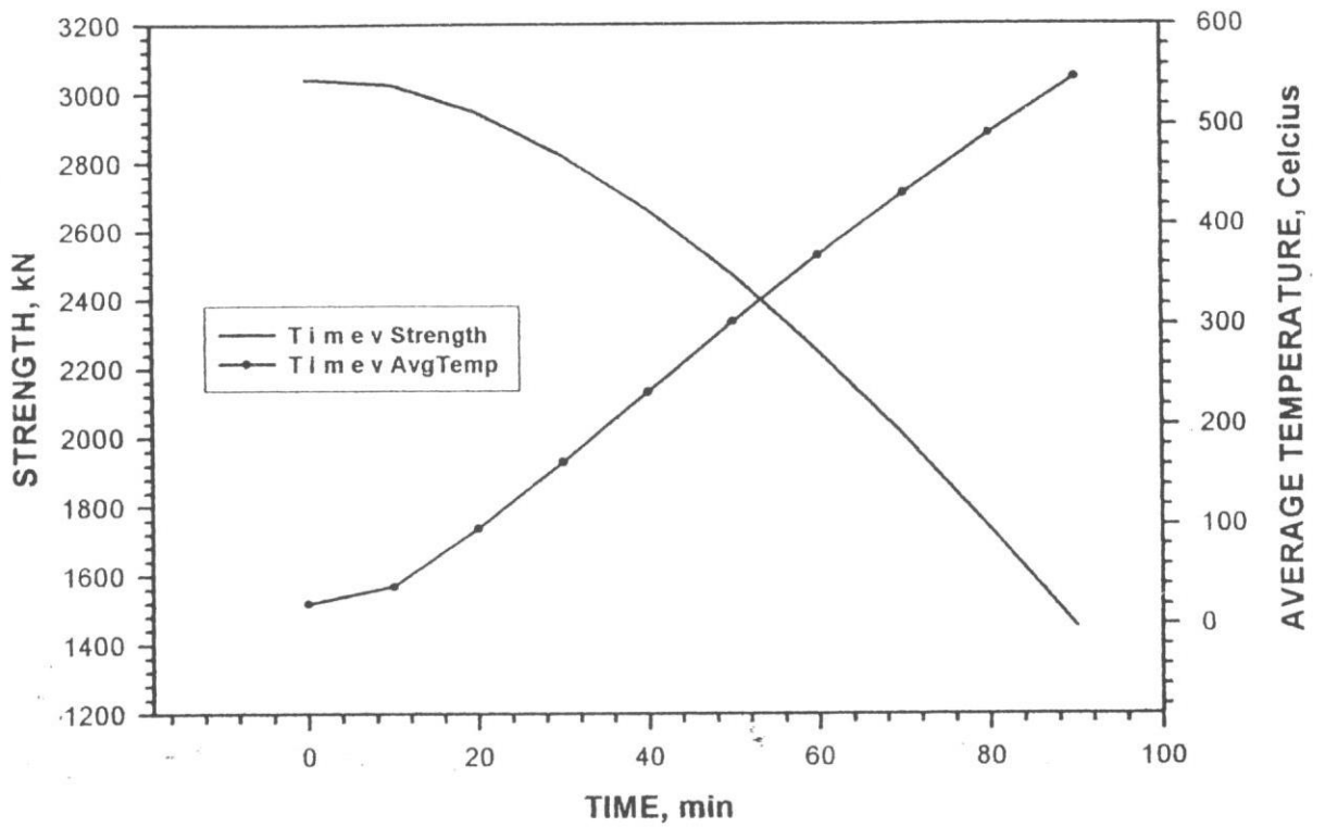
Fig. 15 Column FS4
