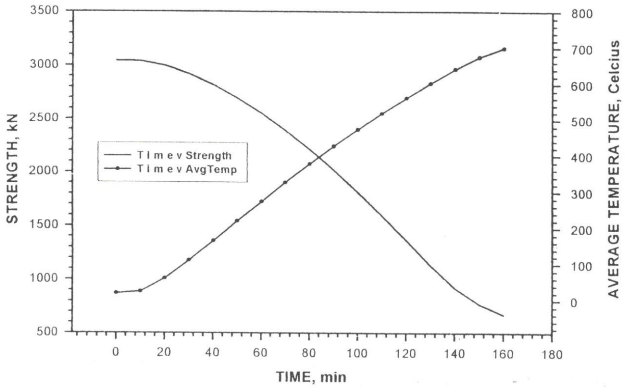
Fig. 13 Column FS2
