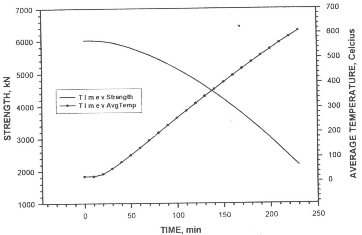
Fig. 16 Column FS5
